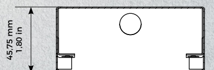
Unterputzgehäuse
