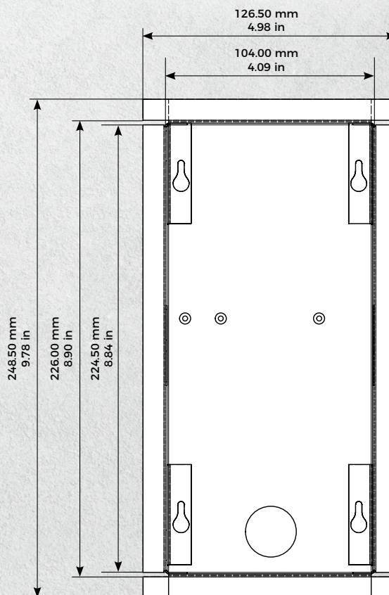
Unterputzgehäuse
