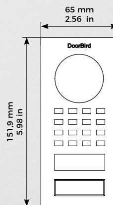
Frontblende
