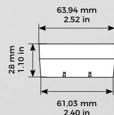
Montagerückgehäuse
